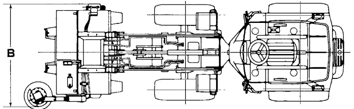
■ 寸法図
